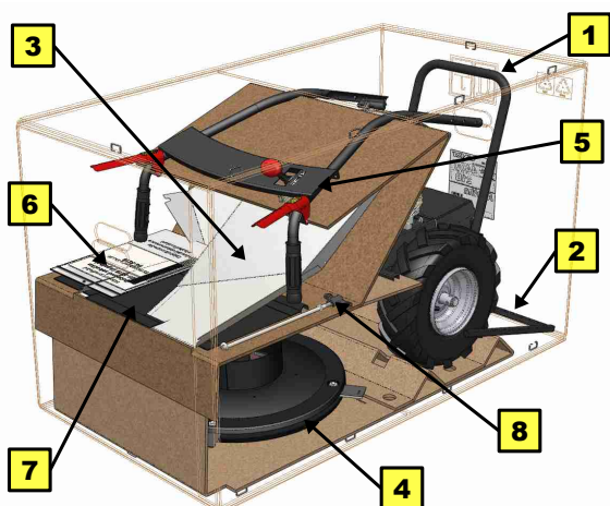
Obr. 1: Vybalení stroje
