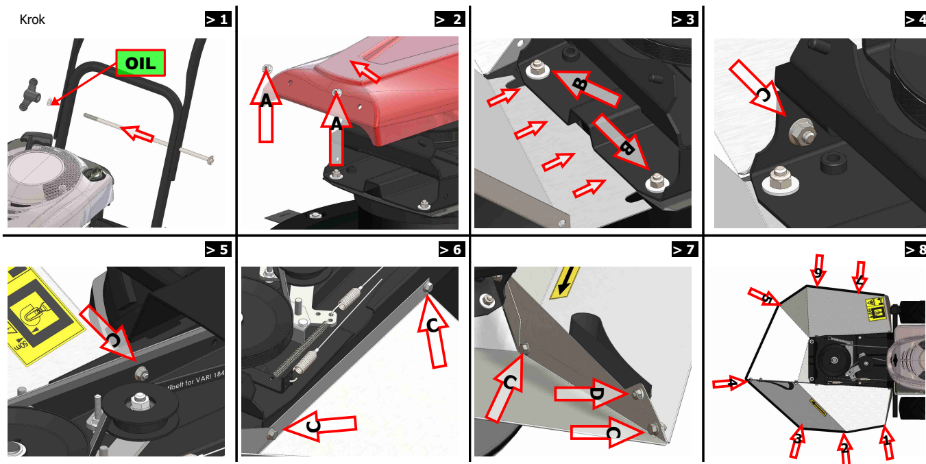
Obr. 3: Sestavení stroje
